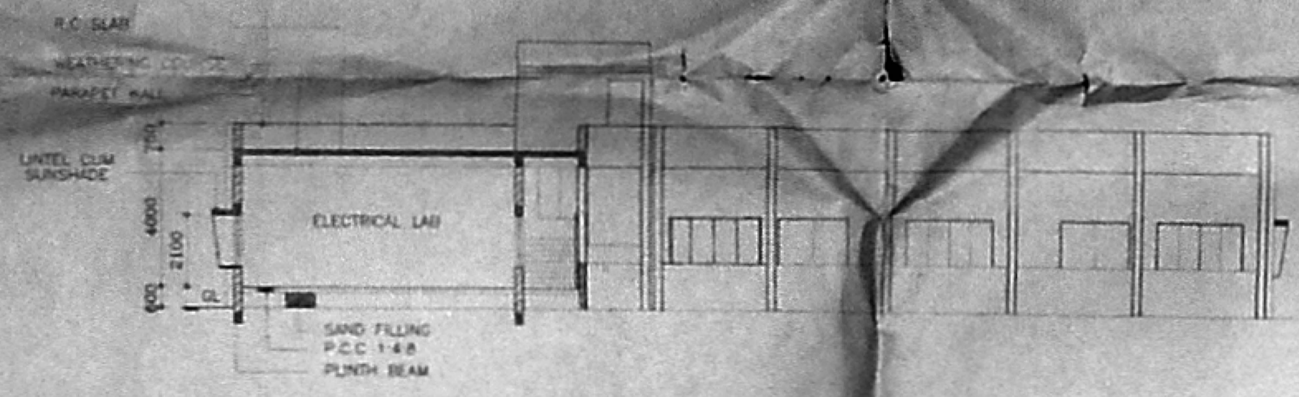
SECTION A-A
